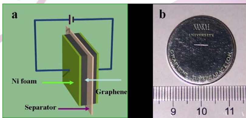
图 4、基于石墨烯的高性能超级电容器
